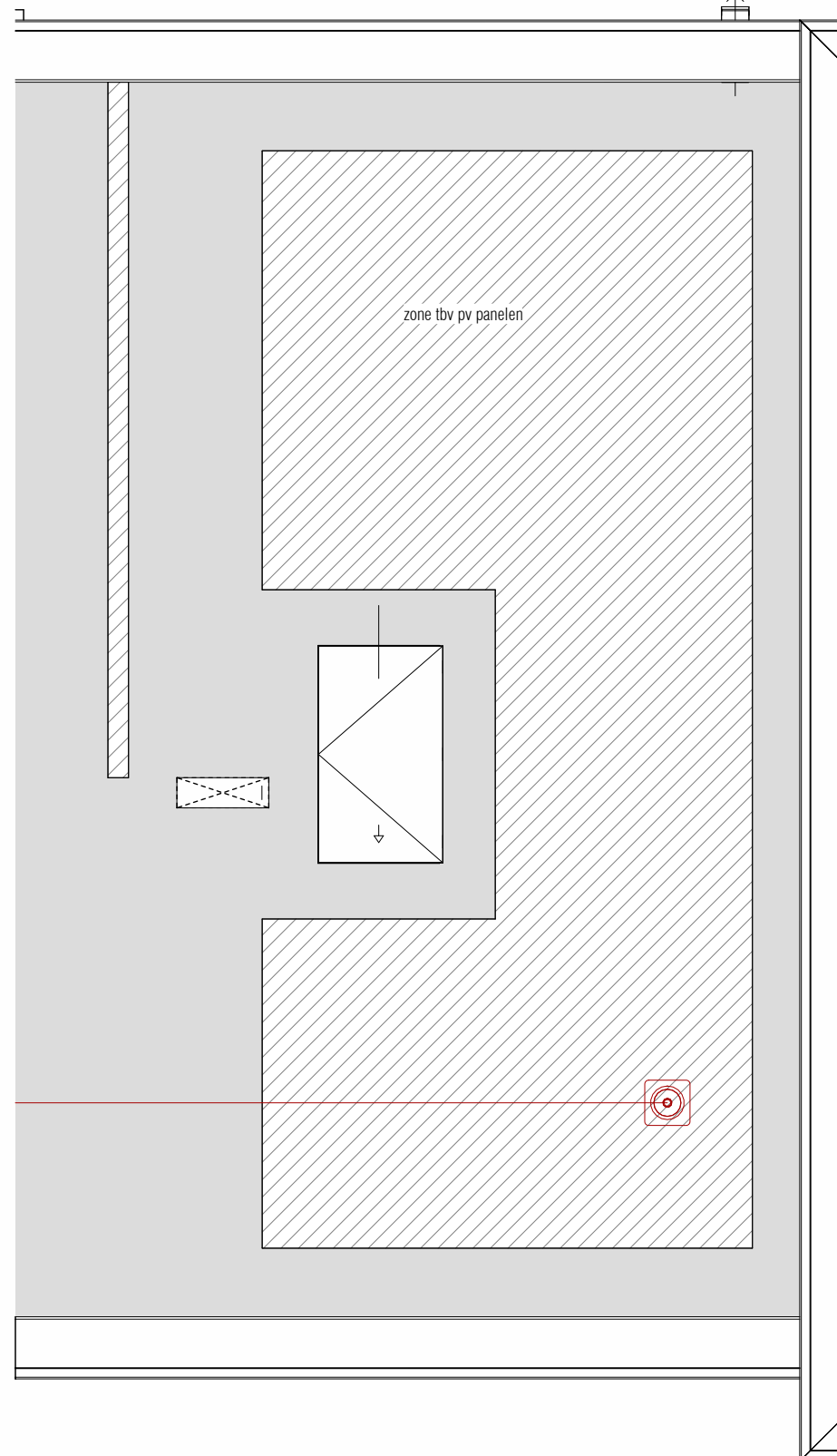
dak verdieping 1 : 50
