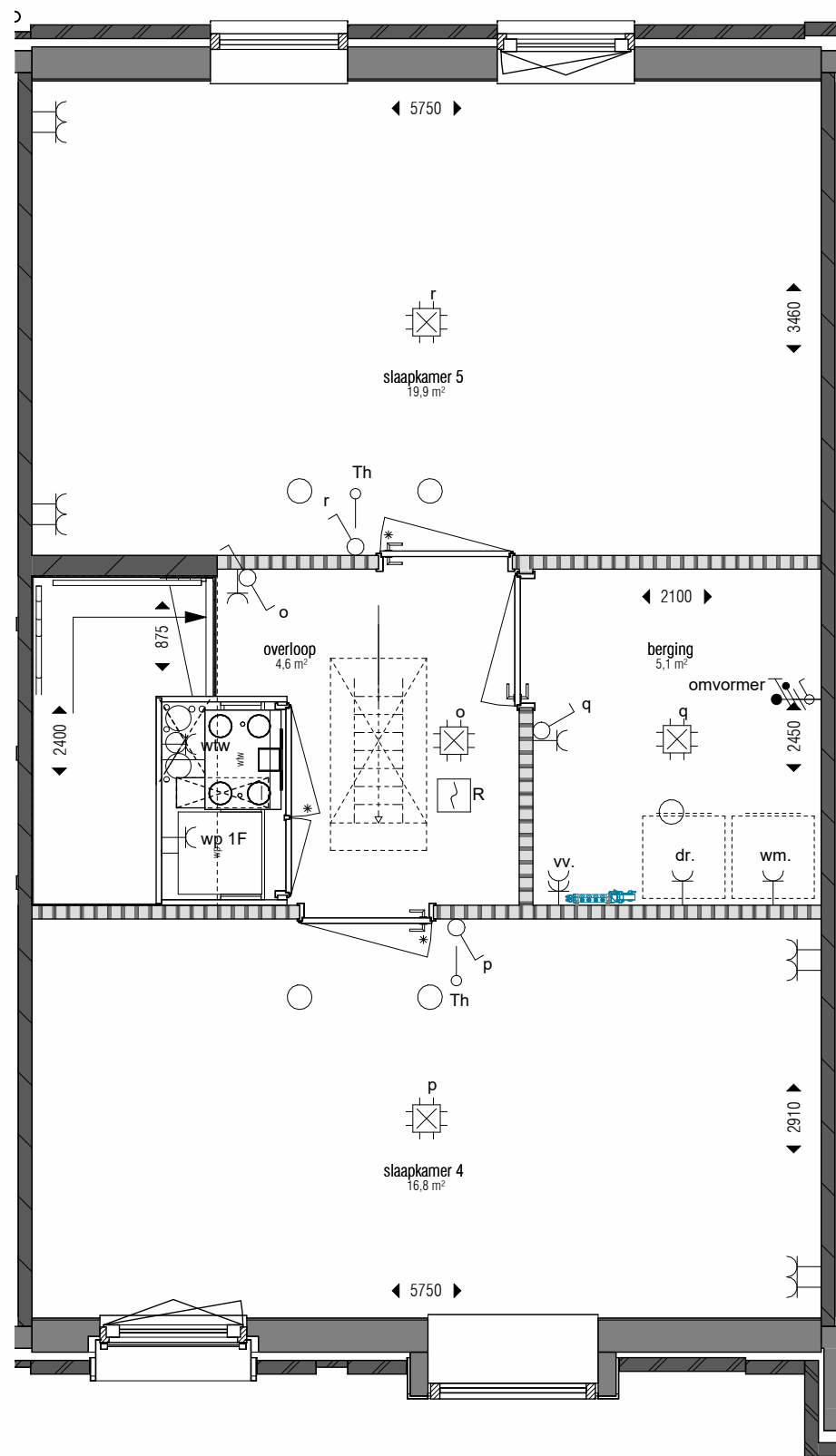
tweede verdieping 1 : 50
