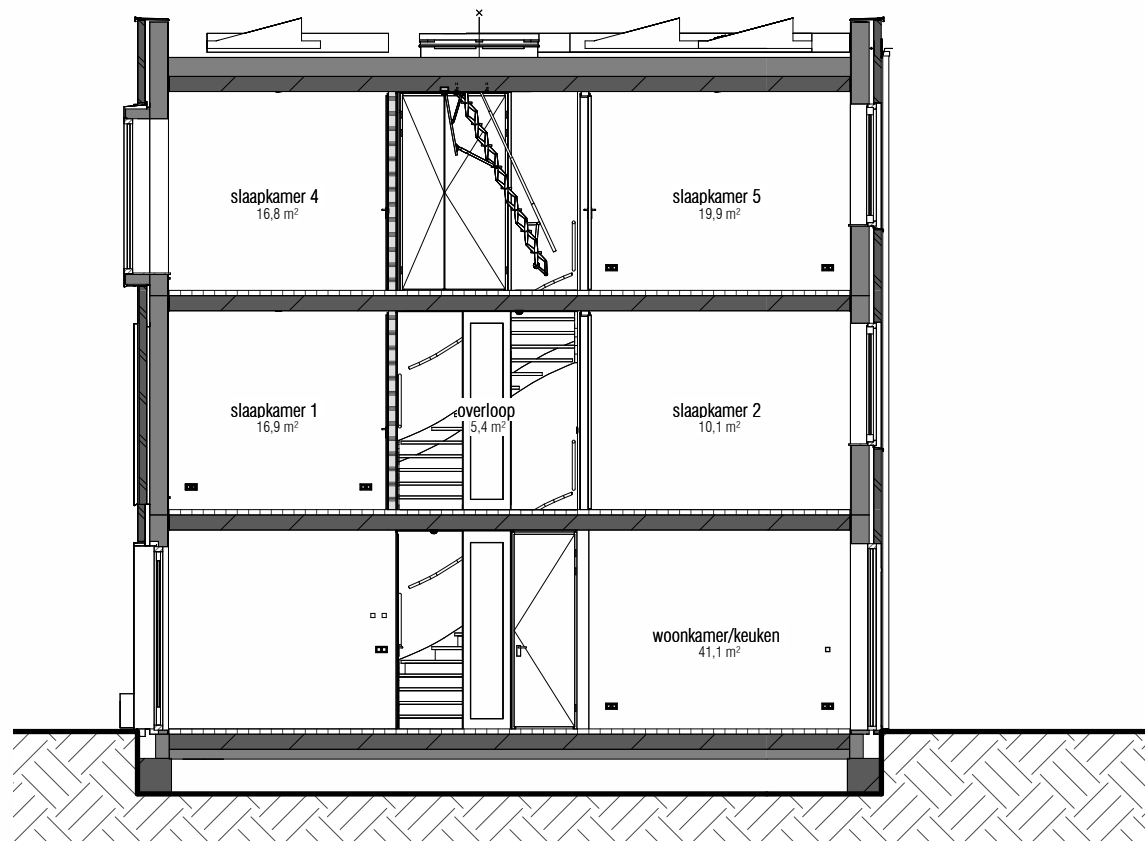
doorsnede 1 : 100
