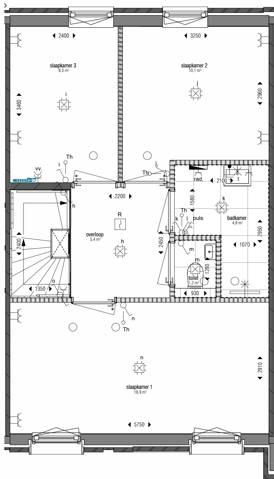
eerste verdieping 1 : 50
